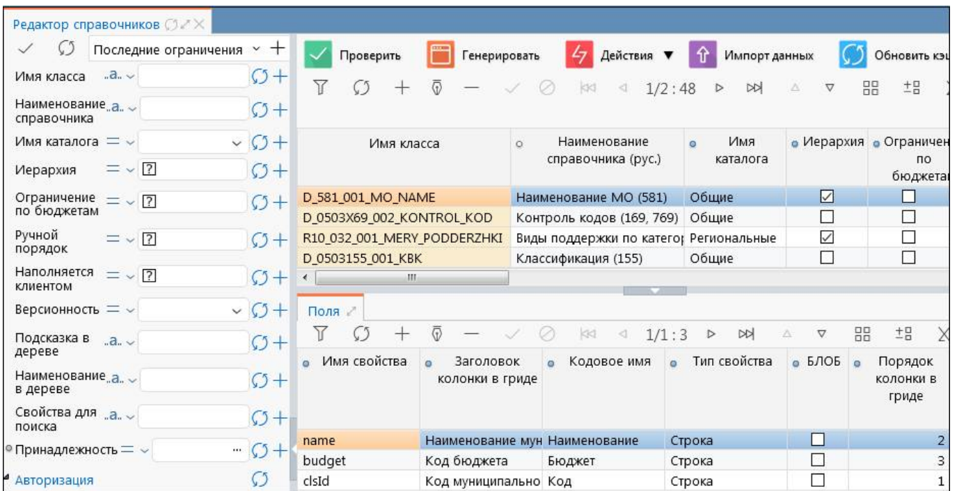
Рисунок 36 – Интерфейс «Редактор справочников»
