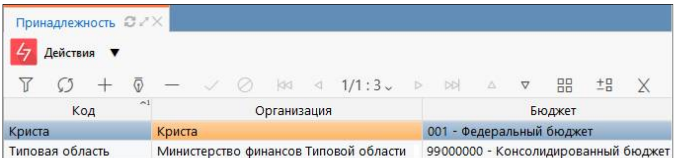
Рисунок 14 – Интерфейс «Принадлежность»
