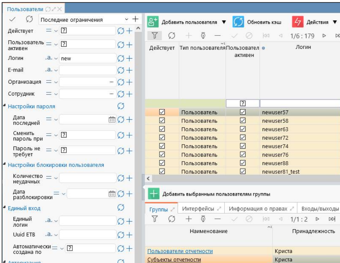
Рисунок 7 – Интерфейс «Пользователи»
